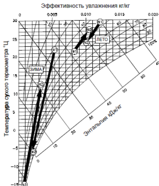
Теплообменник гигроскопический
