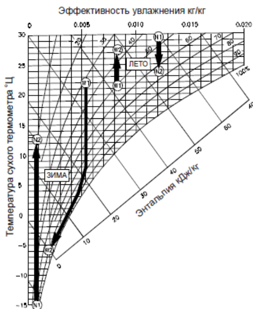
Теплообменник негигроскопический
